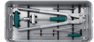
Siebkorb für Helixes .....MP-W85-141 Edelstahl
